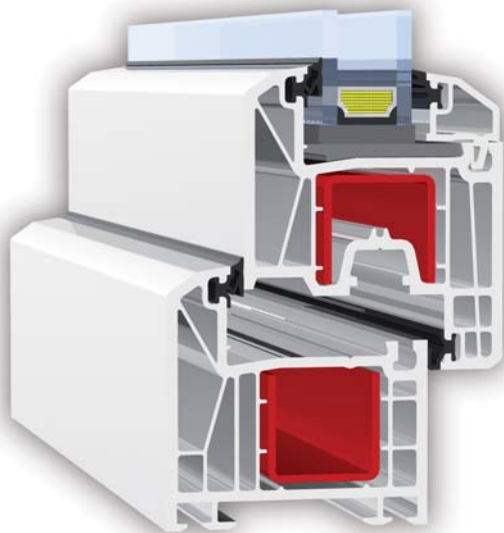
5-Kammer-Anschlagdichtungssystem mit 70mm Bautiefe
