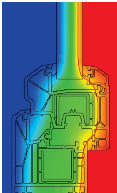
Wärmedämmung: Das Temperaturbild zeigt den optimierten Verlauf der sothermenkurven.
